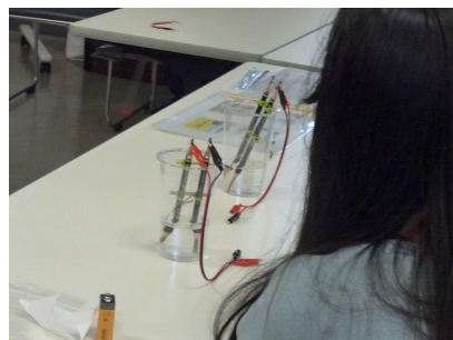
作った電池
